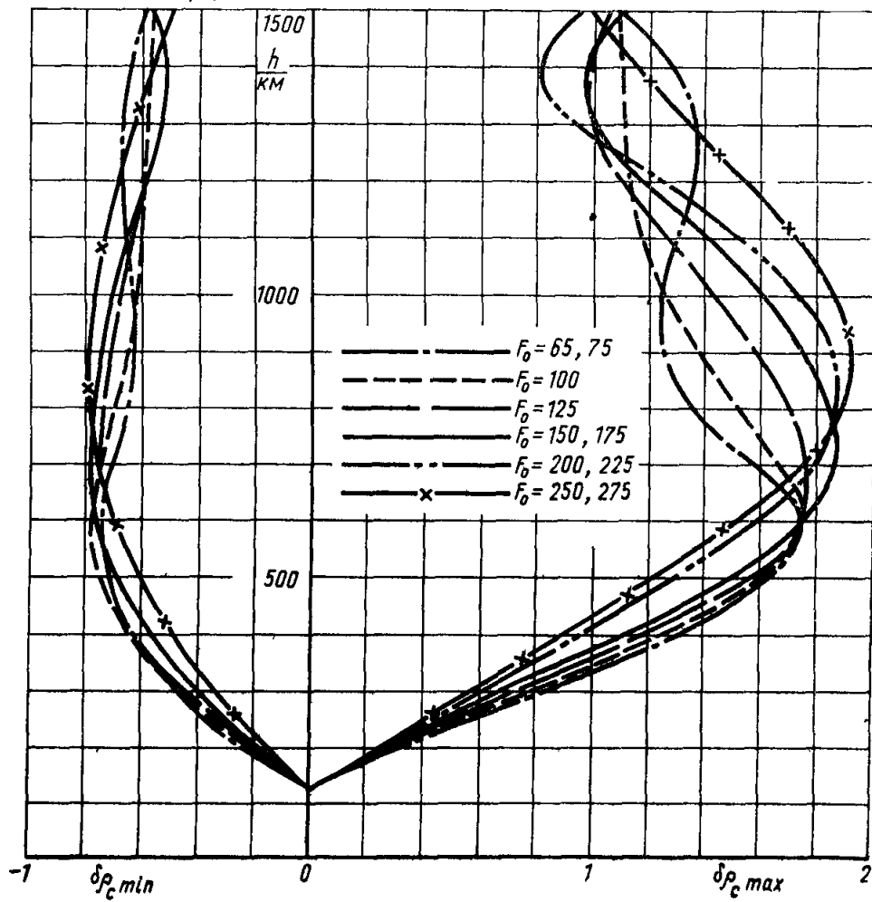
Зависимость величины предельных относительных отклонений плотности атмосферы от высоты в диапазоне от 120 до 1500 км
