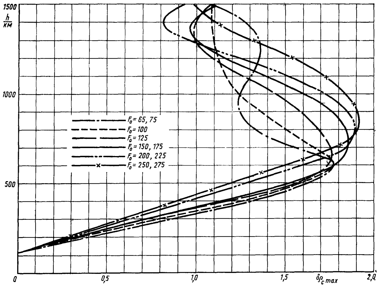
Зависимость максимального относительного отклонения \delta\rho_c \max от высоты в диапазоне от 120 до 1500 км
