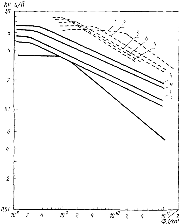
Зависимость коэффициента равноценности радиационного воздействия от величины флюенса протонов СКЛ
