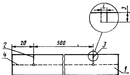
1—образец; 2—первый надрез; 3—второй надрез; 4—шов
