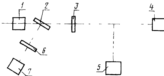
Блок-схема установки для определения чувствительности измерительных приборов
