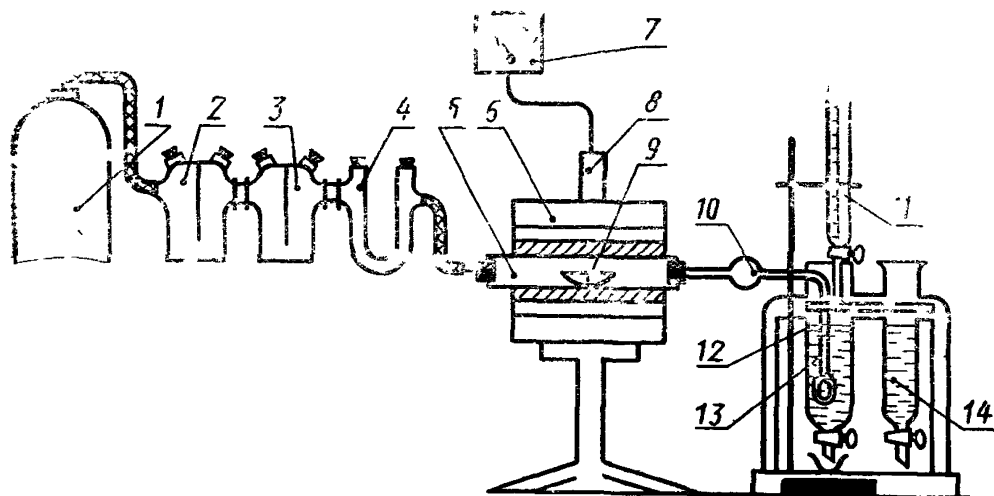
Установка для определения содержания серы
