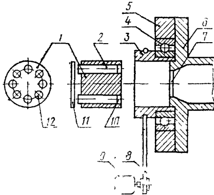
1—кассета; 2—пробка; 3—штулки; 4—подшипник; 5—муфта; 6—мишениная камера; 7—мишень; 8—привод; 9—электродвигатель; 10—пробы и образцы сравнения; 11—крышка; 12—ячейки
