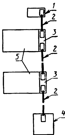
Цепочная конфигурация многокрейтовой системы КАМАК на основе магистрали ветви
