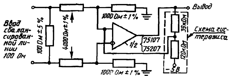
Пример приемника с гистерезисом, дополненным внешними резисторами
