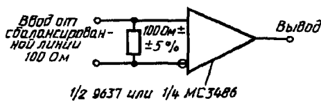
Пример дифференциального приемника
