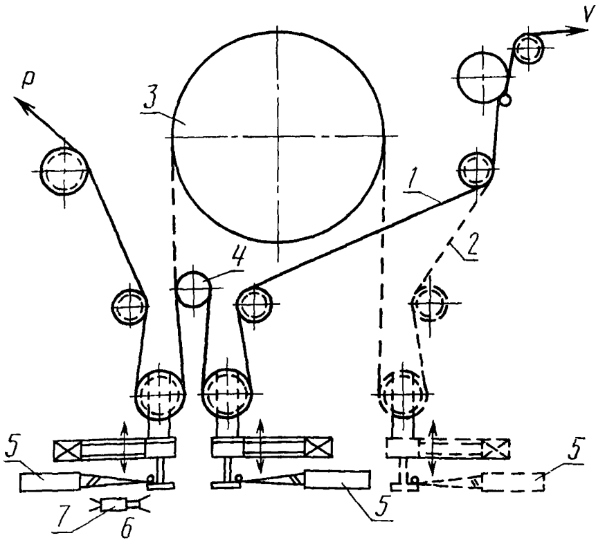
Аппаратура для определения коэффициента динамического трения
