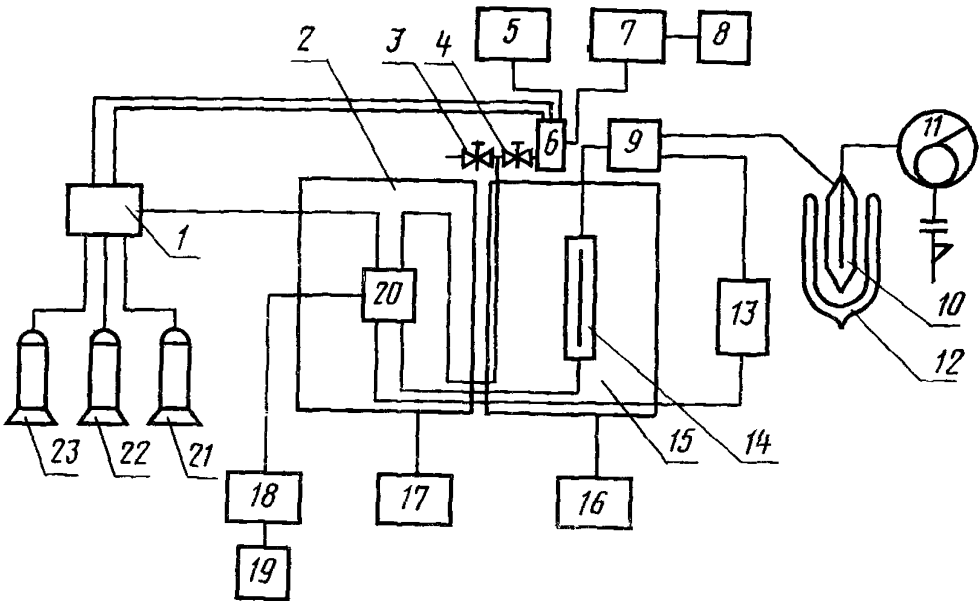
Блок-схема хроматографической установки
