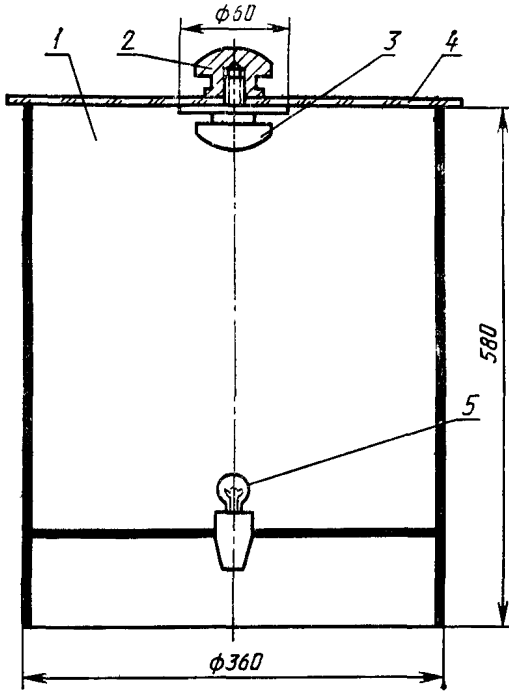
1—корпус; 2—ручка; 3—винт; 4—крышка; 5—источник освещения
