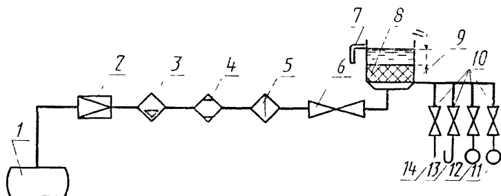
1—источник сжатого воздуха; 2—редукционный клапан; 3—влагомаслоотделитель; 4—осушитель; 5—фильтр; 6—кран точной регулировки; 7—сливная трубка для установки уровня жидкости над образцом; 8—испытуемый образец; 9—держатель для крепления образцов; 10—кран; 11—манометр Мо 0,4 МПа по ГОСТ 6521—72; 12—манометр Мо 0,16 МПа по ГОСТ 6521—72; 13—U-образный манометр, заполненный водой; 14—микроманометр ММН-2400(5)—0,6 ГОСТ 11161—84.
