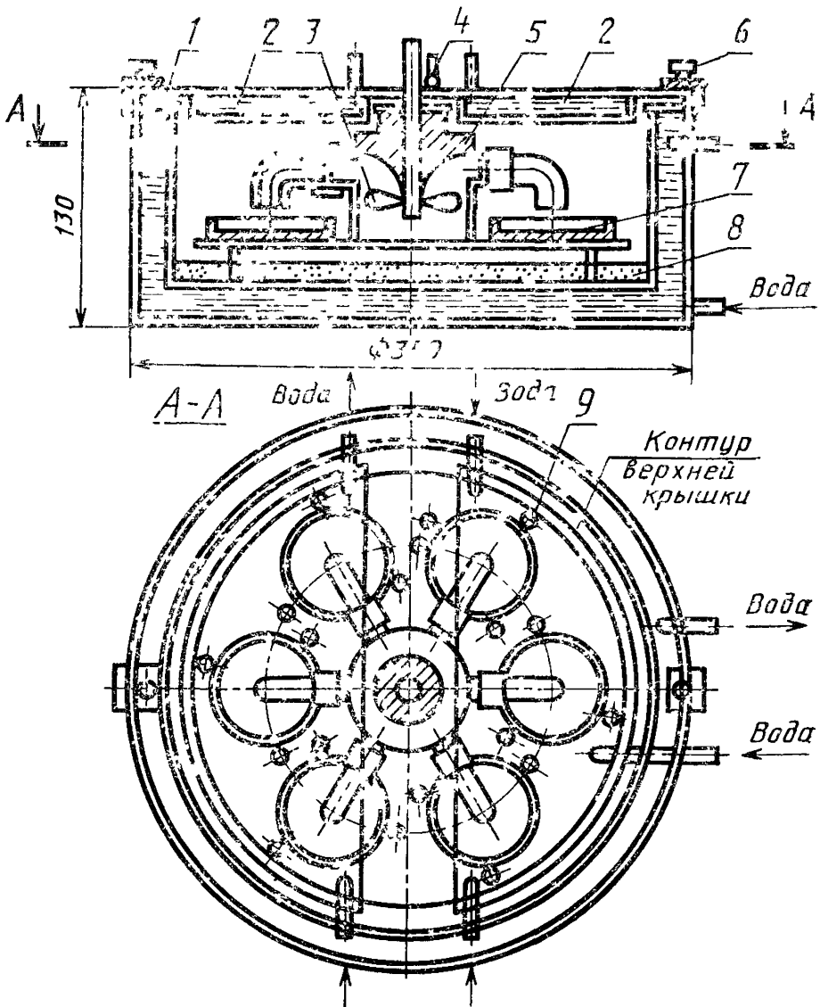
1 — сосуд с двойными стенками, 2 — крышка, состоящая из двух частей, 3 — перепеллер, 4 — термометр, 5 — бронзовый подшипник, 6 — винтовые зажимы, 7 — бюксы, 8 — насыщенный раствор сульфата калия, 9 — штифты
