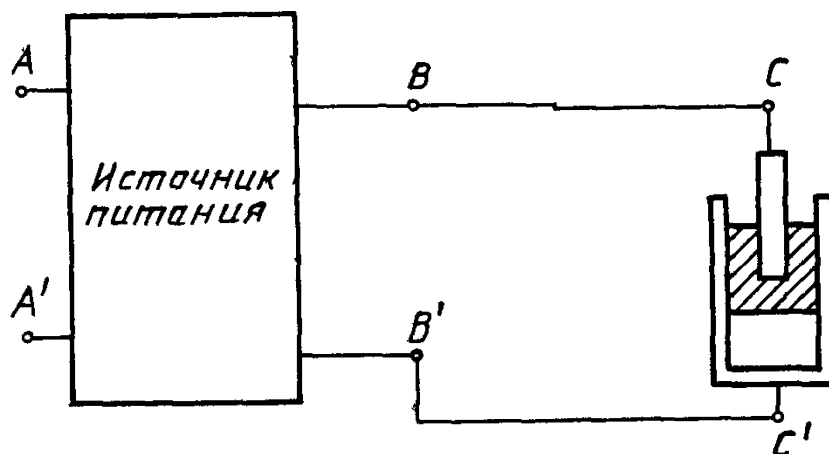
Схема электропитания печи
