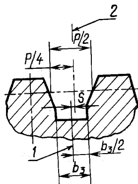
Положение оси симметрии канавки: 1 — действительное, 2 — номинальное
