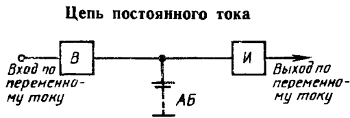
В —выпрямитель; И —инвертор; АБ —аккумуляторная батарея Черт. 1
