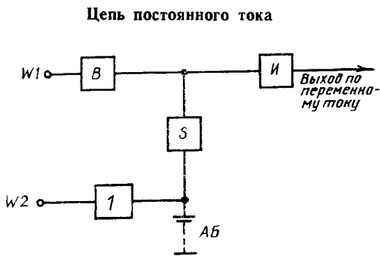
1 — выпрямитель зарядки батареи; W1 , W2 — входы по переменному току; S — блокирующий диод, тиристор или коммутирующее устройство Черт. 2
