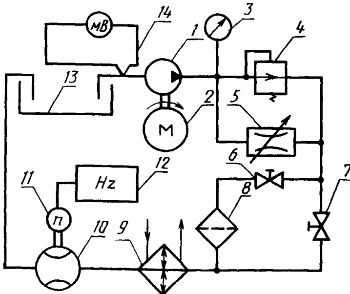
1—испытываемый насос, 2—электродвигатель; 3—манометр; 4—предохранительный клапан; 5—дрозсель; 6, 7—вентили; 8—фильтр; 9—теплообменник; 10—расходомер; 11—индукционный датчик; 12—частотомер; 13—бак с рабочей жидкостью; 14—термопара
