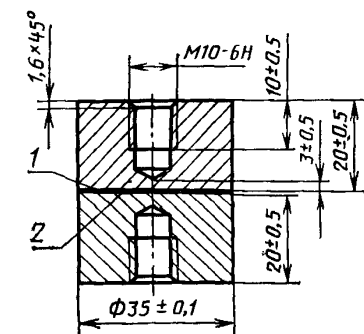
1—испытуемое покрытие; 2—клеевой шов
