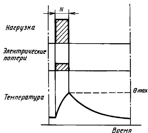
Кратковременный режим Типовой режим S2
