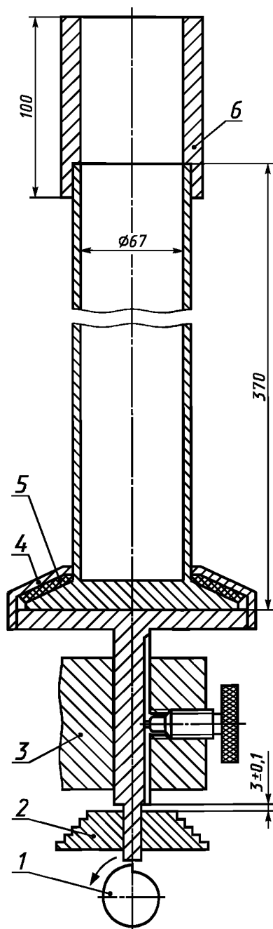
Аппарат для уплотнения механическим методом
