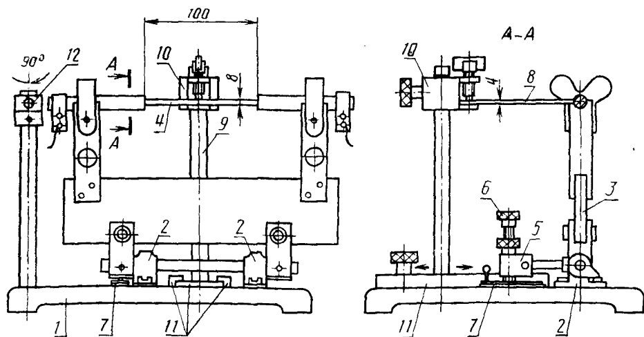
1—опорная плита; 2—подшипники; 3—держатель; 4—накаливаемый стержень; 5—противоповоз; 6—опорный винт; 7—поворотная пластина; 8—испытуемый образец; 9—держатель образца; 10—зажим; 11—подвижное основание; 12—поворотный металлический стержень
