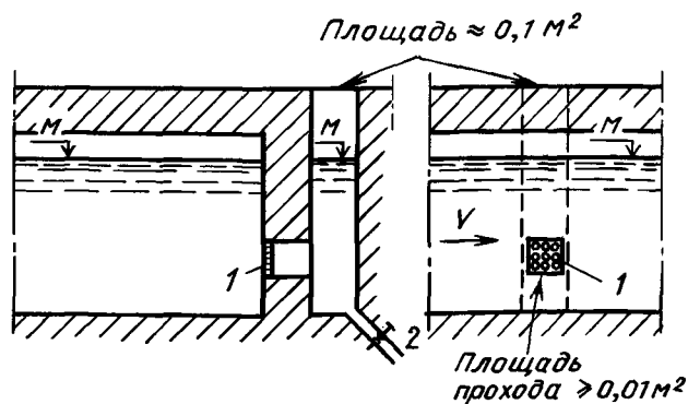
Измерительный колодец
