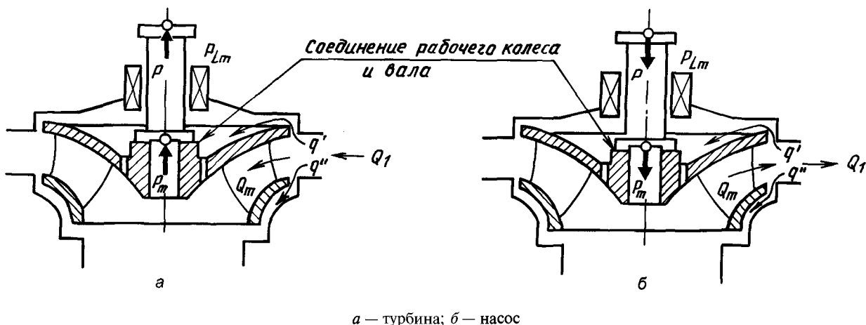
Схема для определения баланса мощности и расхода
