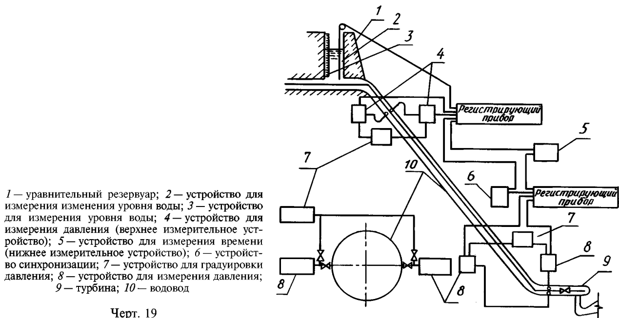
Схема измерения расхода методом «гидроудара» с помощью раздельных диаграмм
