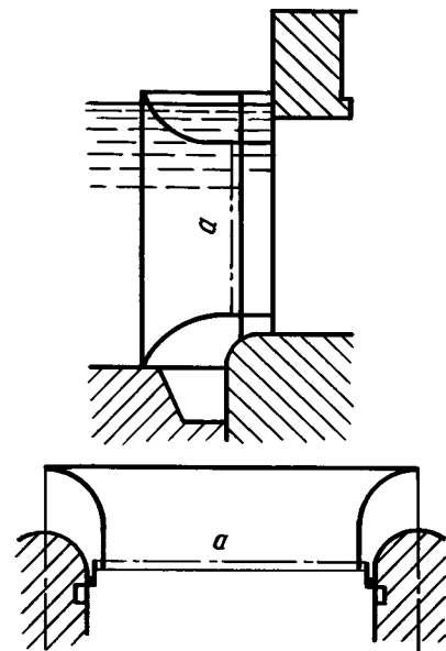
a — измерительное сечение
