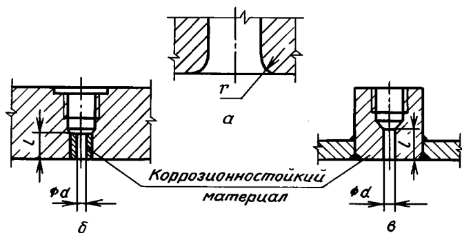
Примеры отверстий для отбора давления
