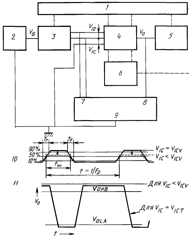
Измерение пускового синфазного входного напряжения
