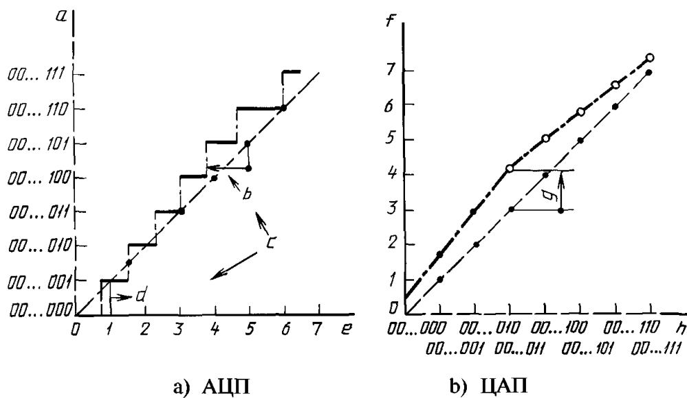
a — цифровые выходные коды; b — на ступени 00...101 ( -1\frac{1}{4} LSB); c — полная погрешность; d — на ступени 00...001 ( +1\frac{1}{2} LSB); e — аналоговые входные величины (LSB); f — аналоговые выходные величины (LSB); g — общая погрешность на ступени 00...011 ( +1\frac{1}{8} LSB); h — цифровые входные коды
