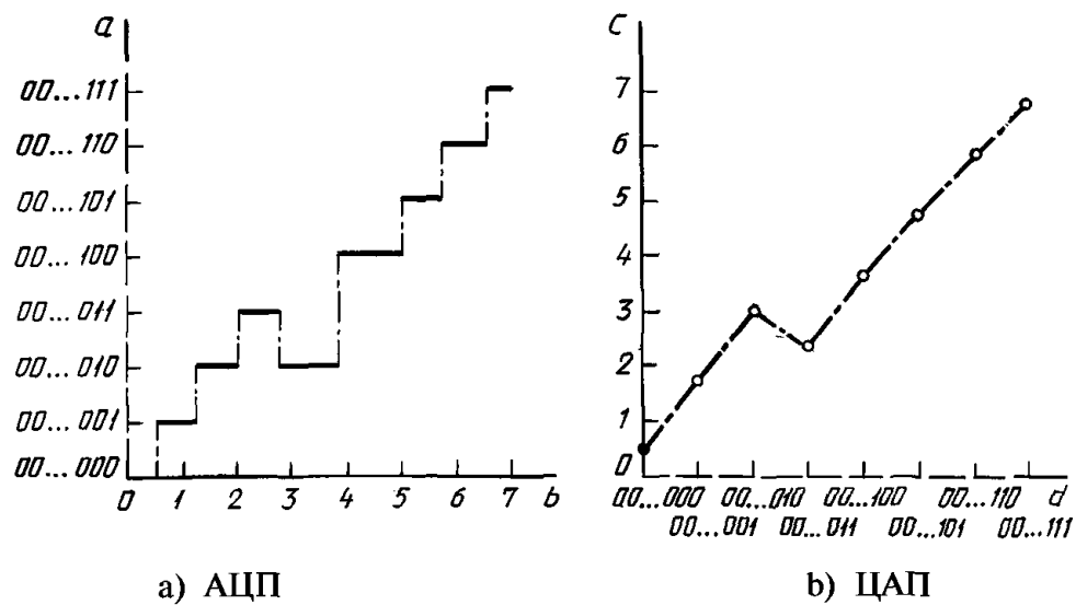
a — цифровые выходные коды; b — аналоговые входные величины (LSB); c — аналоговые выходные величины (LSB); d — цифровые входные коды
