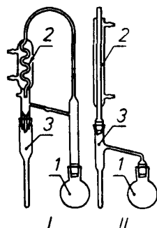
Рисунок 1 — Установка для прямого объемного метода определения влаги
