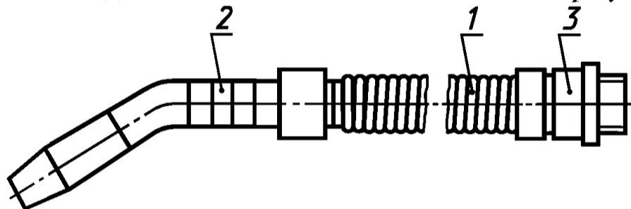
1 — рукав; 2 — наконечник; 3 — патрубок
