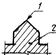
1 — радиус кривизны опоры (макс. 0,25 мм); 2 — опора
