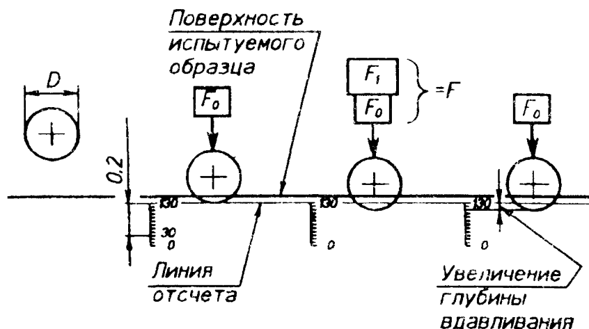
Рисунок 4 — Испытание на твердость методом вдавливания
