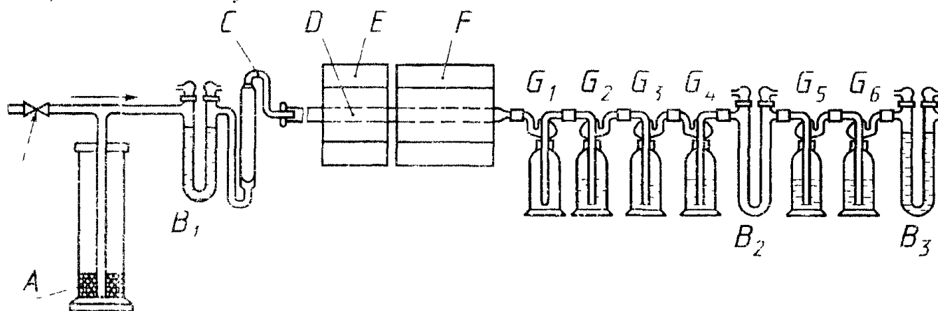
1 - цилиндр с ртутью; B_1 , B_2 , B_3 - U-образные трубки; C - реометр; D - трубка из кварца; E - электропечь, обеспечивающая температуру нагрева 800–900 °С; F - электропечь, обеспечивающая температуру нагрева 400–450 °С; G_1 – G_6 - склянки Дрекслея
