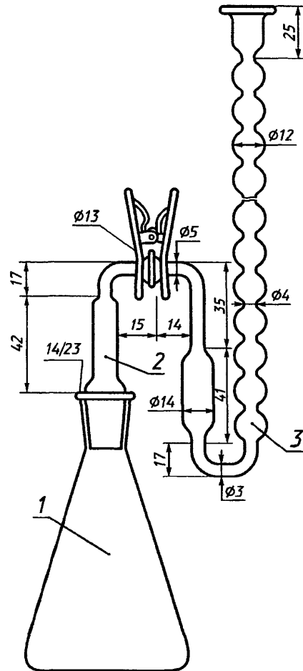
1 — коническая колба; 2 — соединительная трубка; 3 — абсорбер
