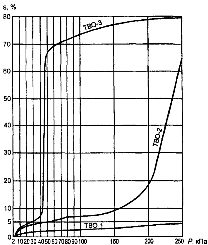
Рисунок Б.1 — Диаграммы \epsilon = \epsilon(P)
