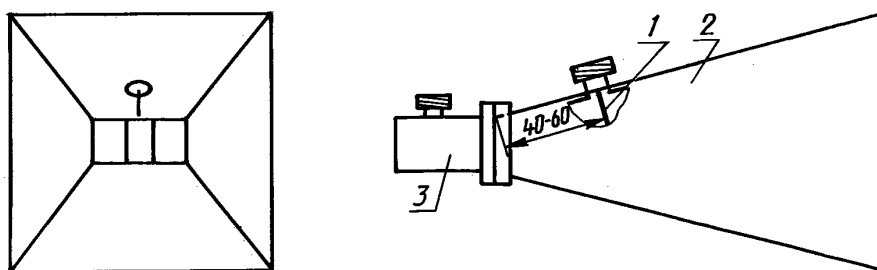
Приемопередающая антенна
