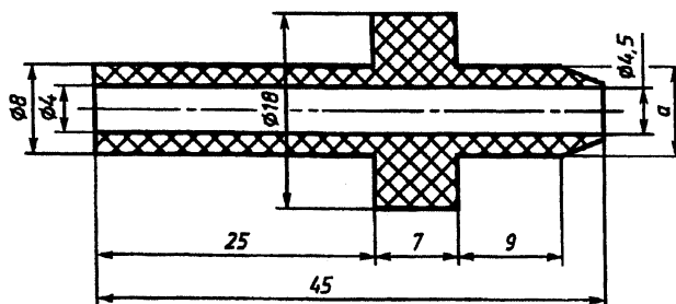
a — диаметр 5, 6, 7, 8 мм в зависимости от размера лабиринтового уплотнения
