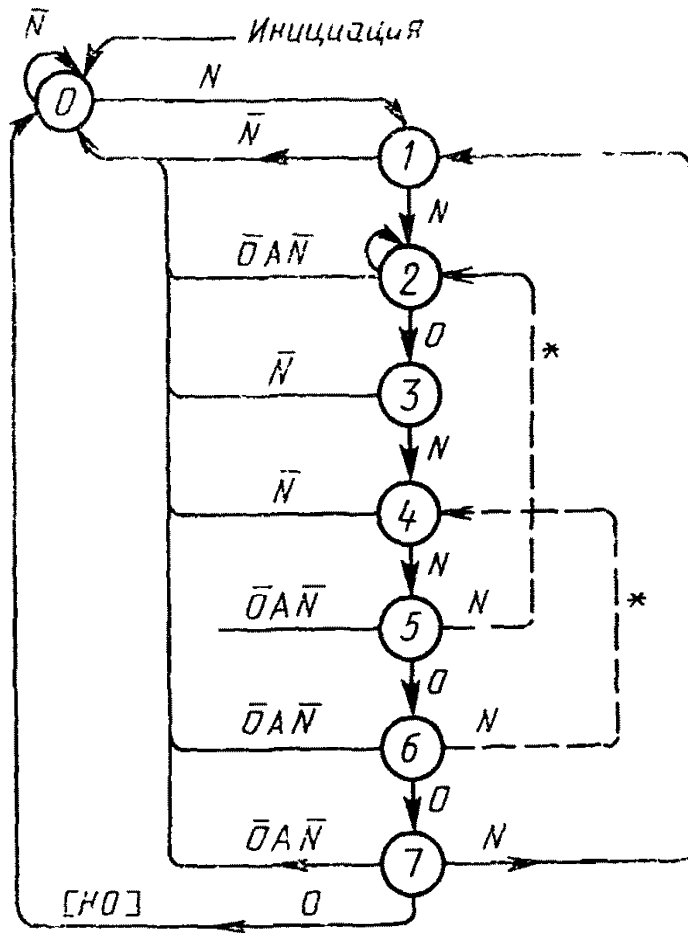
Конечный автомат обнаружения молч/раб
