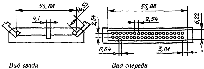
Розетка одинарного интерфейсного соединителя
