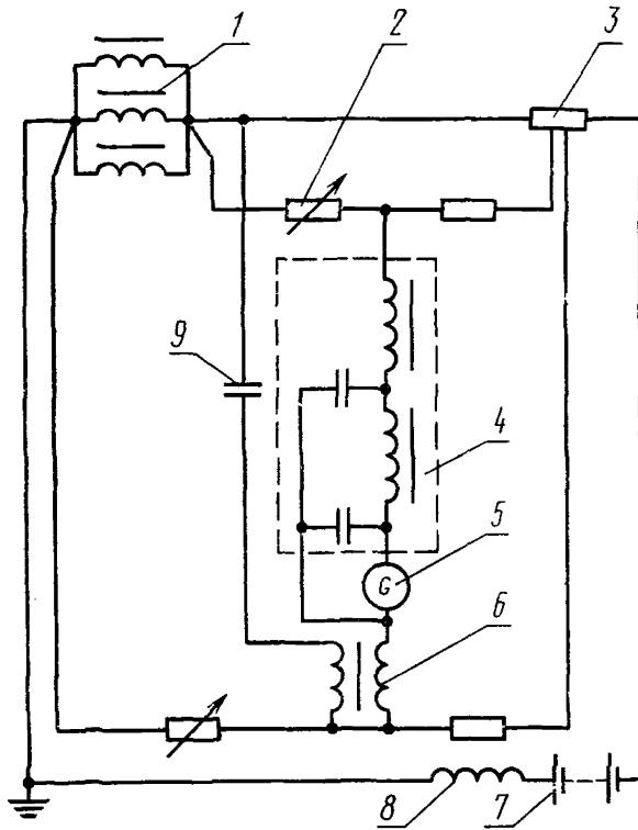
1—измеряемая обмотка; 2—регулируемый резистор; 3—резистор; 4—фильтр; 5—гальванометр; 6—трансформатор компенсирующий; 7—аккумуляторная батарея; 8—дрозсель; 9—разделительный конденсатор
