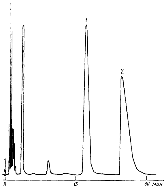
Хроматограмма образца фенхелевого масла
