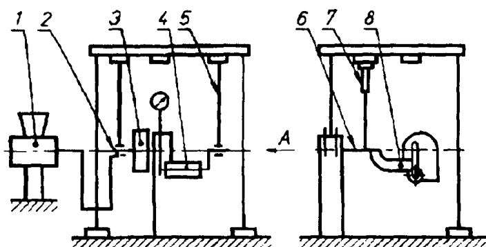
1 — мясорубка; 2 — поводок; 3 — редуктор; 4 — двигатель; 5 — стойка; 6 — планка; 7 — индикатор часового типа; 8 — рычаг Стенд для испытания мясорубки
