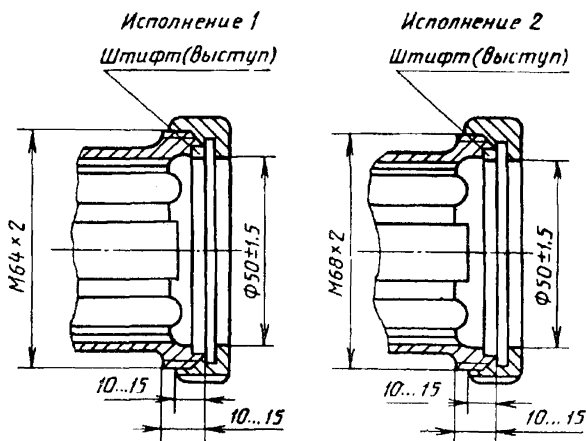
Рисунок 5 — Накидная гайка
