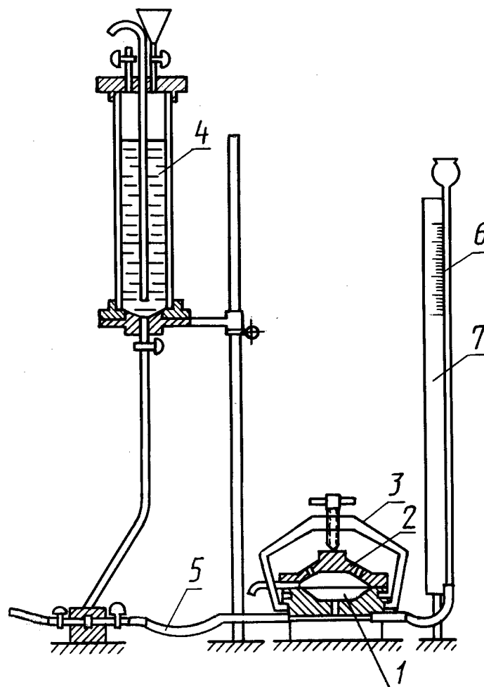
1 — резервуар для воды; 2 — кольцевой зажим; 3 — струбцина; 4 — стеклянный цилиндр; 5 — резиновые трубки; 6 — водяной манометр; 7 — штатив
