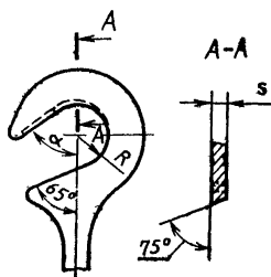
Нож противорежущий
