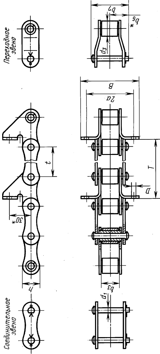
Тип 2. Исполнение 2
