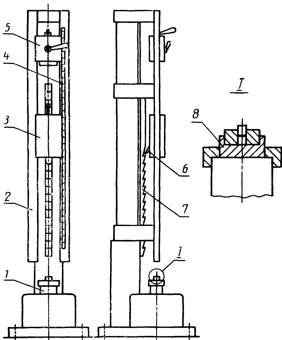
Схема копра
