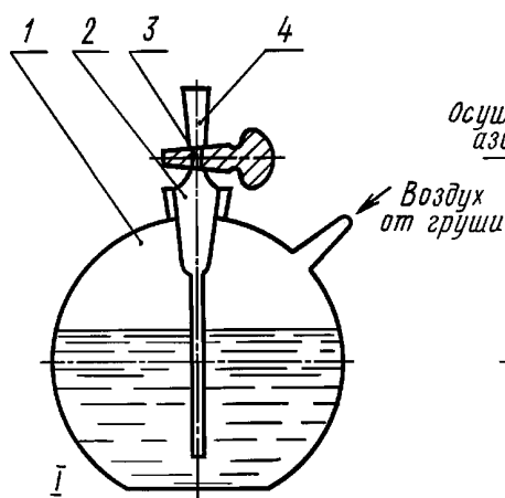
I-положение крана-дозатора при заполнении из колбы
