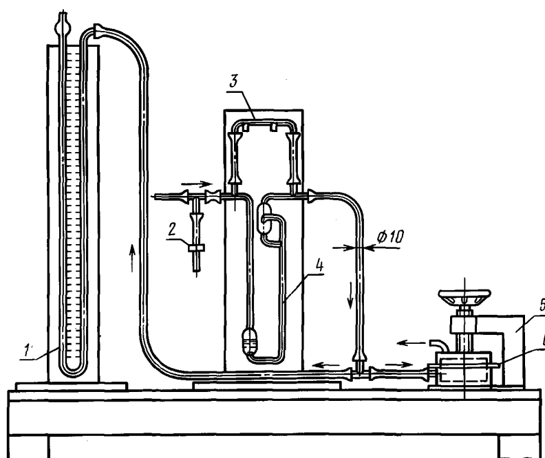
Схема установки для определения сопротивления пластин потоку воздуха
