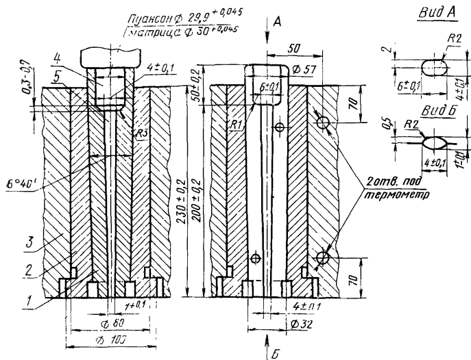
1—полуматрица; 2—стакан матрицы; 3—обойма матрицы; 4—загрузочная камера; 5—камера стрелки
