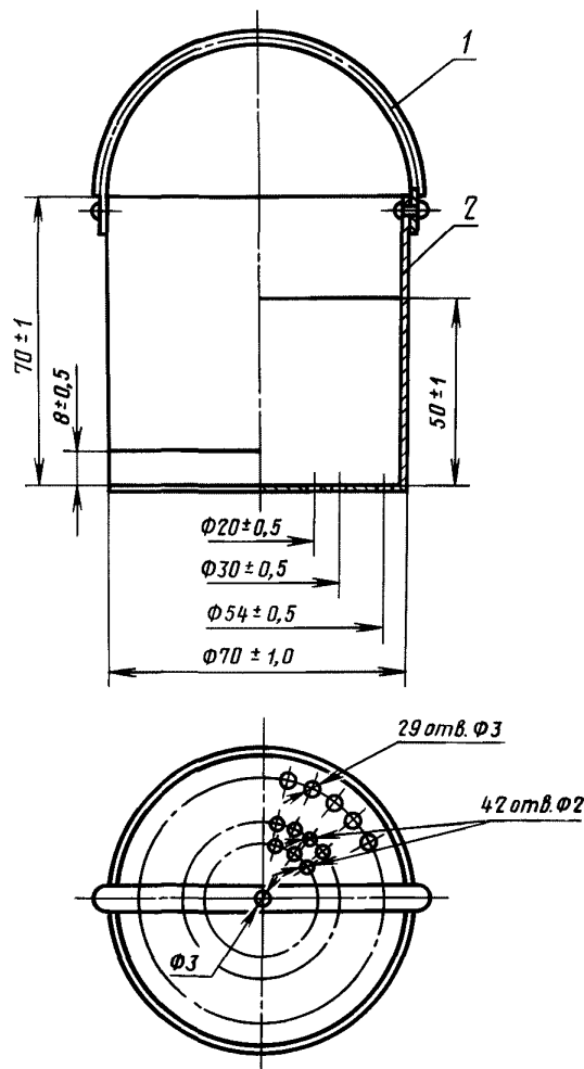
1 — ручка; 2 — корпус
