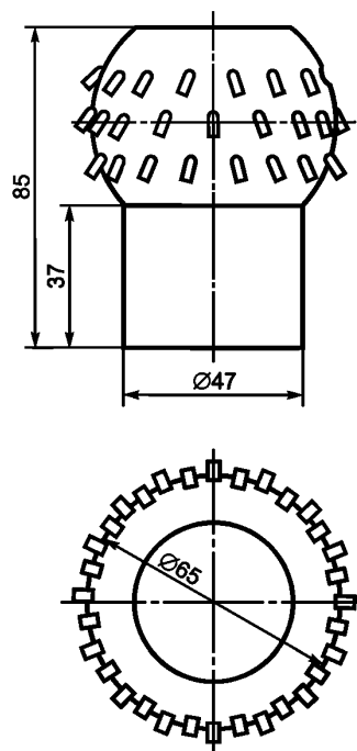
Защитный колпачок
