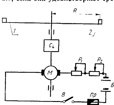
1—крестовина, 2—стойка для крепления анемометров, C_4 —счетчик частоты вращения крестовины, M —двигатель; P_1 , P_2 —реостаты, B —аккумуляторная батарея; B —выключатель, Пр —предохранитель
