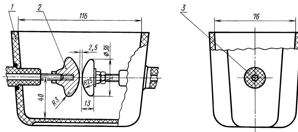
Измерительная ячейка для определения пробивного напряжения
