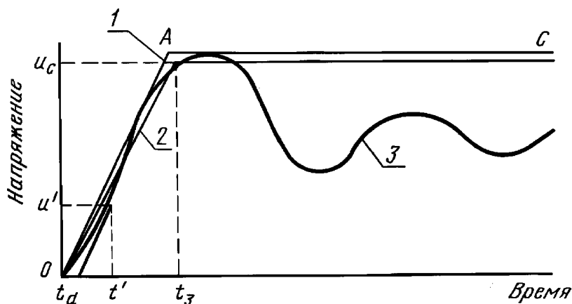
Построение огибающей ПВН, определяемого двумя параметрами
