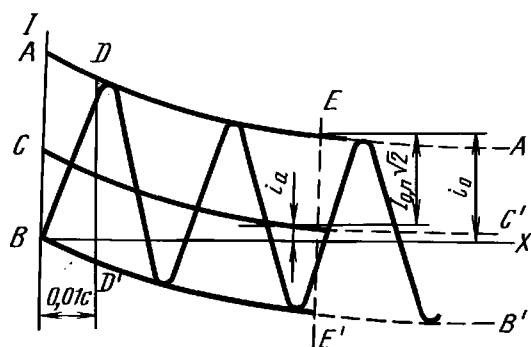
Периодическая и аperiodическая составляющие тока короткого замыкания
