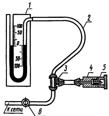
1 — ртутный манометр; 2 — шланг; 3 — тройник; 4 — патрон; 5 — пробка; 6 — кран
