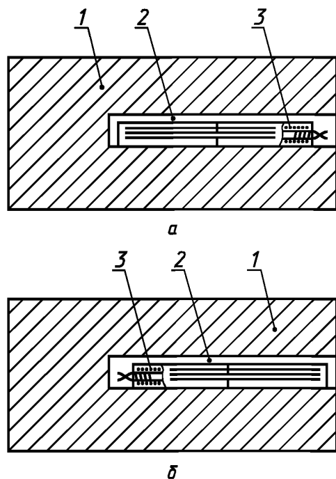
a — прямое инициирование; б — обратное инициирование 1 — канальная мортира; 2 — сквозной канал; 3 — заряд ВВ с электродетонатором
