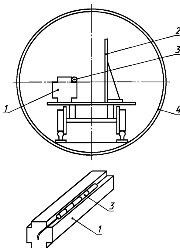
1 — угловая мортира; 2 — отражательная стенка; 3 — испытуемый заряд ВВ; 4 — шпрек
