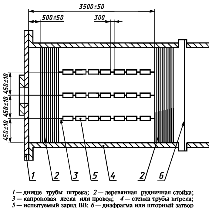
Рисунок 4 — Схема испытания взрыванием рассредоточенных зарядов
